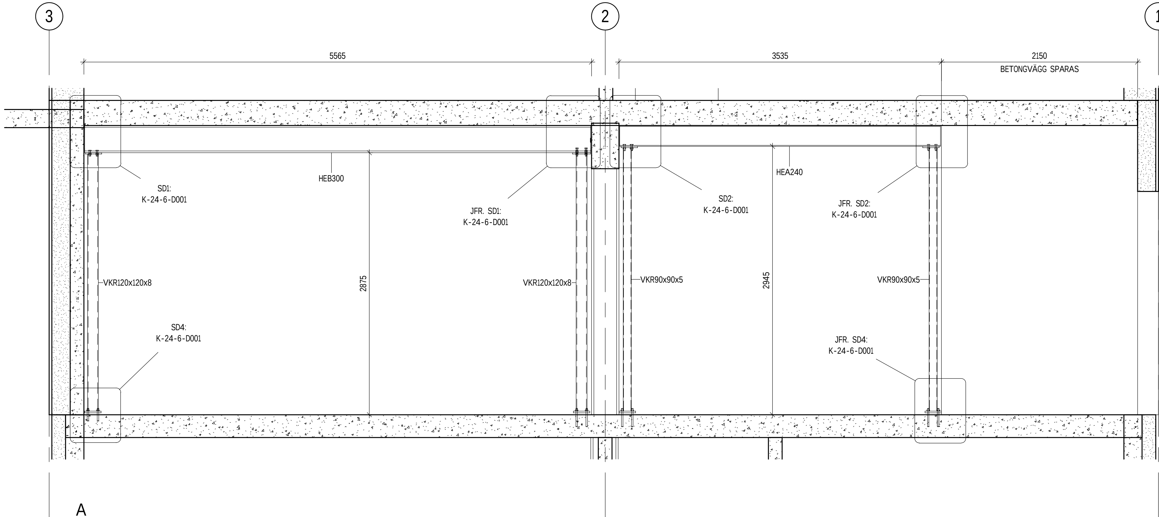
A 1 : 25
